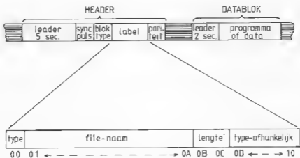
Afb. 6-1 Indeling van de cassetteband
